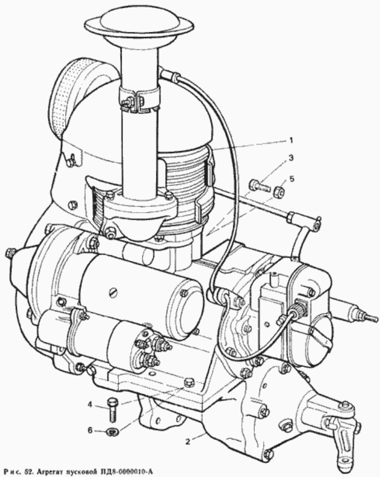
Рис. 52. Агрегат пусковой ПД8-0000010-А
